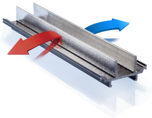
Bildunterschrift: insulbar LEF: Das Wärmedämmprofil nutzt eine Low-E-Folie die Wärmestrahlung reflektiert. Außen- und Innenschalen von Metallrahmen für Fenster, Türen und Fassaden werden dadurch optimal thermisch getrennt.
