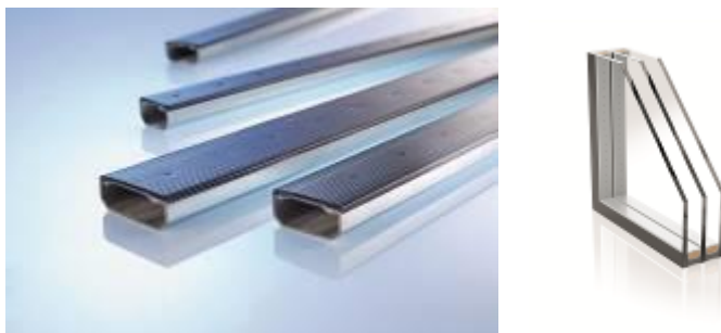
Photos 3 + 4 : Les intercalaires Thermix de chez Ensinger procurent l'effet « warm edge » dans le vitrage isolant – certifié pour les maisons passives. Photo : Ensinger GmbH
