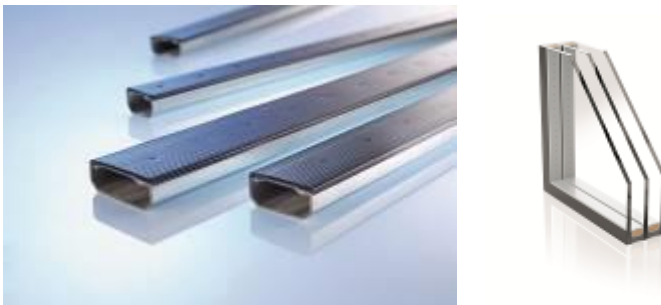
Bild 3 + 4: Thermix Abstandhalter von Ensinger sorgen für die "warme Kante" in der Isolierverglasung - Passivhaus zertifiziert. Bild: Ensinger GmbH
