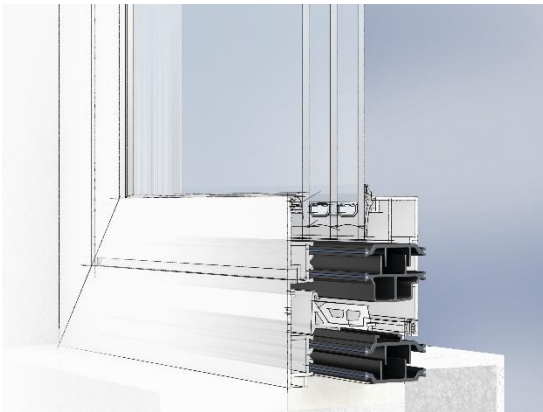
Abb. 1: So einfach kann thermische Trennung im Metallrahmen sein: Ensinger bietet im insulbar Standard-Programm fertige Komplettlösungen mit aufeinander abgestimmten Profil-Geometrien in vielen Dämmtiefen an.
